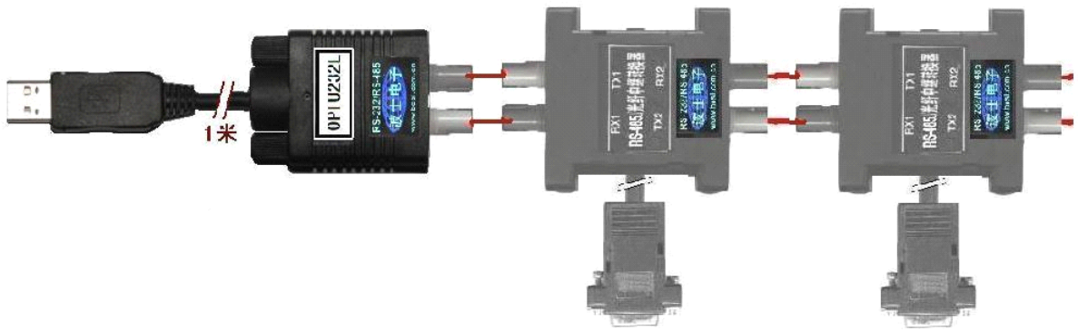
图 2： USB、串口光纤多机通信图
