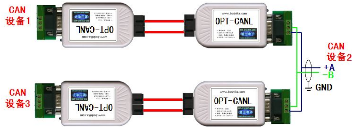
图 3 双纤多机通信
