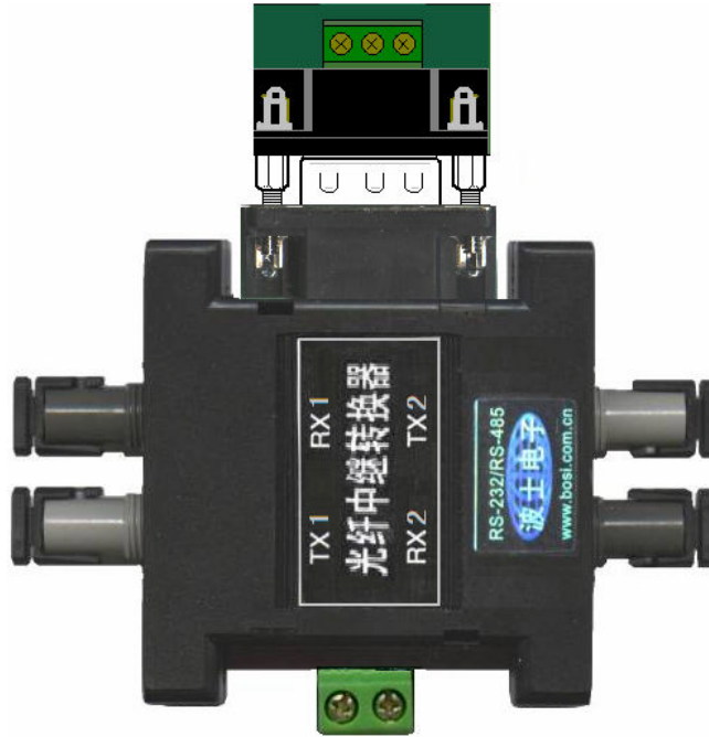
与 OPT-CAN[S]配套的型号为 OPT-CAN-EX[S]的 CAN/光纤中继转换器产品外形图
